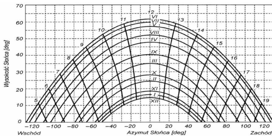
Rys 3.1. Wysokość i azymut Słońca dla 52°N
